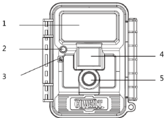
1. IR-LED-es vaku 2. Fényszenzor 3. Mikrofon 4. PIR-szenzor 5. Objektív (mozgásérzékelő)
