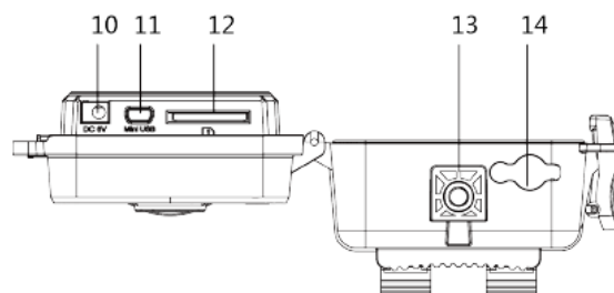
10. 6V-os DC-aljzat 11. USB-aljzat 12. SD-kártya aljzat 13. Szabvány állványmenet
